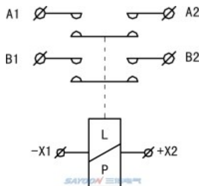
AH二路常开 (DPDT 2NO) A1、A2、B1、B2为触点接线端 -X1、+X2为线圈接线端
