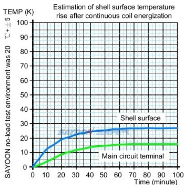
温升曲线图
