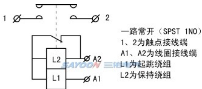
线路原理图
